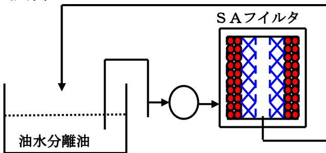
油回収容器 油水分離槽
