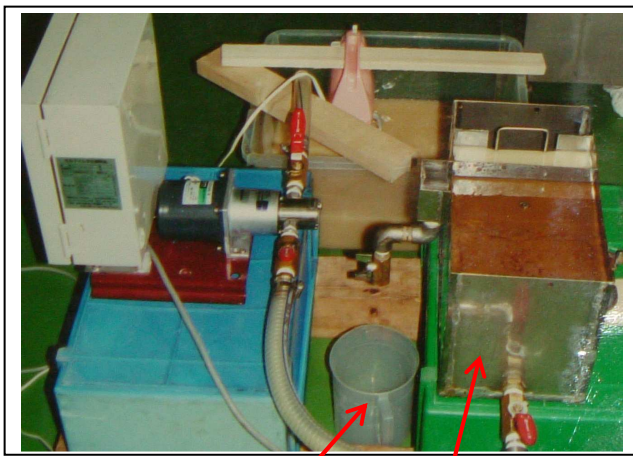
油回収容器 油水分離槽
